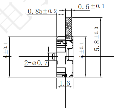
PCB板位置尺寸
