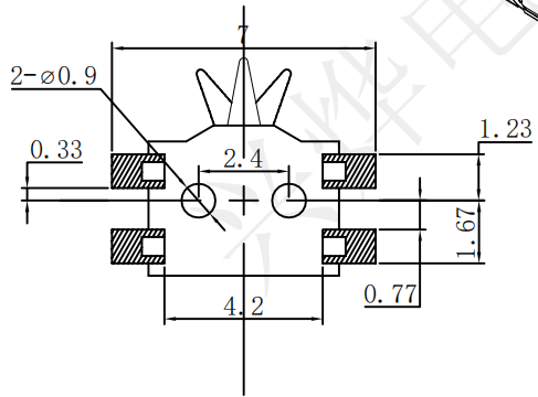
PCB板位置尺寸
