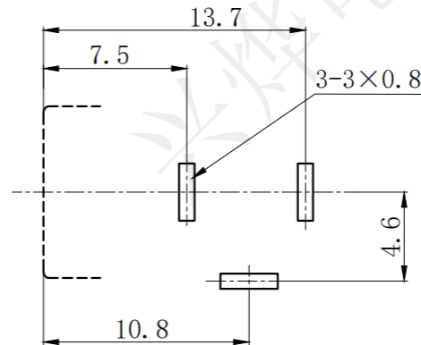
线路板开孔尺寸
