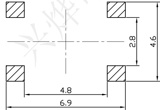
安装参考图
