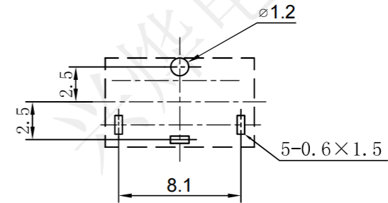
线路板安装示意图
