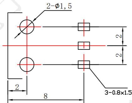
线路板开孔尺寸 P.C.B LAYOUT
